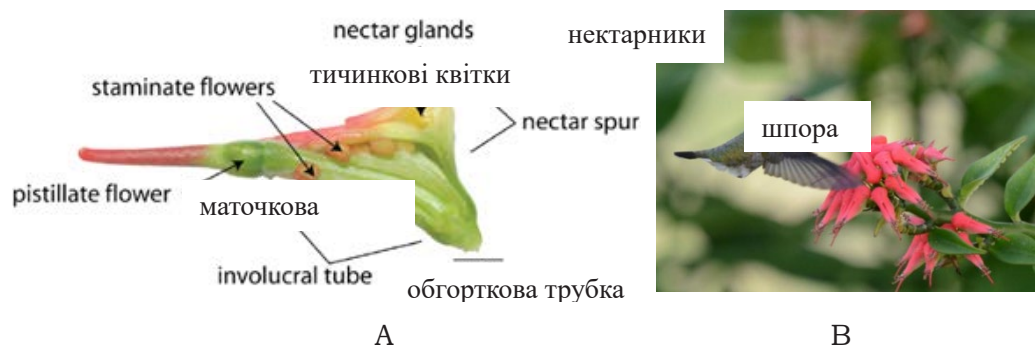
Рис. 11. А – поздовжній середній зріз шпорчастого зигоморфного циатію Euphorbia tithymaloides subsp. padifolia (L.) V.W.Steinm., шпора, що приховує нектарники (Cacho et al., 2010); В – вербеновий колибри Mellisuga minima запилює E. tithymaloides , фото Hans Krause (López-Marmolejo, 2023)
