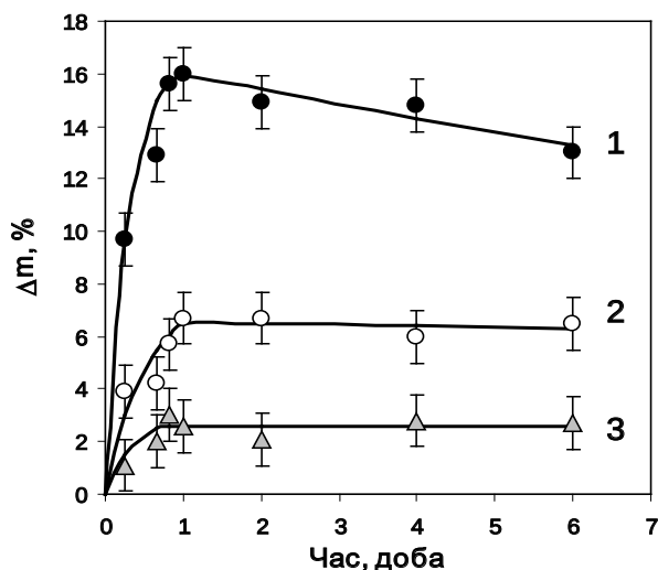
Рис. 1. Зміни ваги вугілля Д (1), Ж (2) та \text{PC}_2 (3) зі збільшенням часу контакту з розчином азотної кислоти
